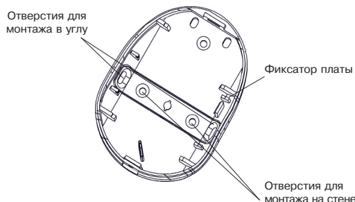
Рисунок 2 — Основание извещателя
