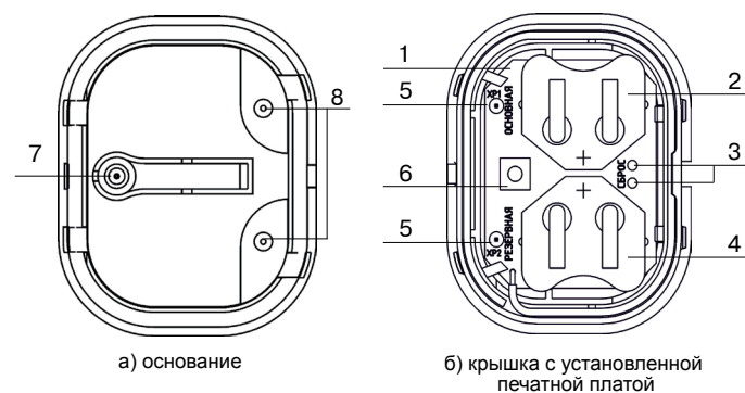
Рисунок 1 – Конструкция извещателя
